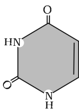
Uracil (Pyrimidine)
