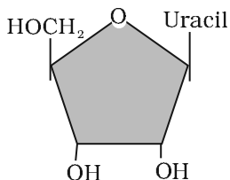
Uridine
